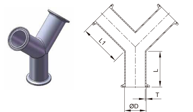
28BMP 90° Y TRUE CLAMP END
